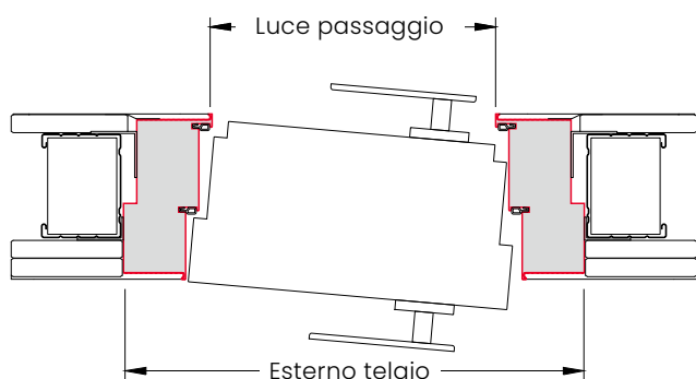
PARTICOLARE APERTURA A TIRARE
