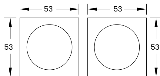
Nicchie di serie. Cromo satinato o lucido
