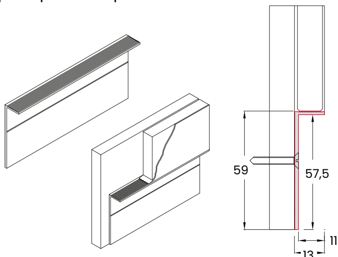
profilo per battiscopa
