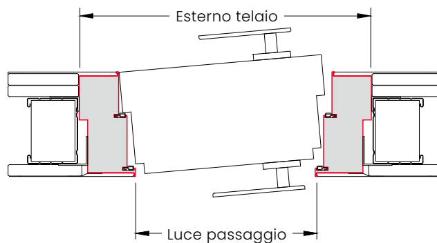
PARTICOLARE APERTURA A SPINGERE
